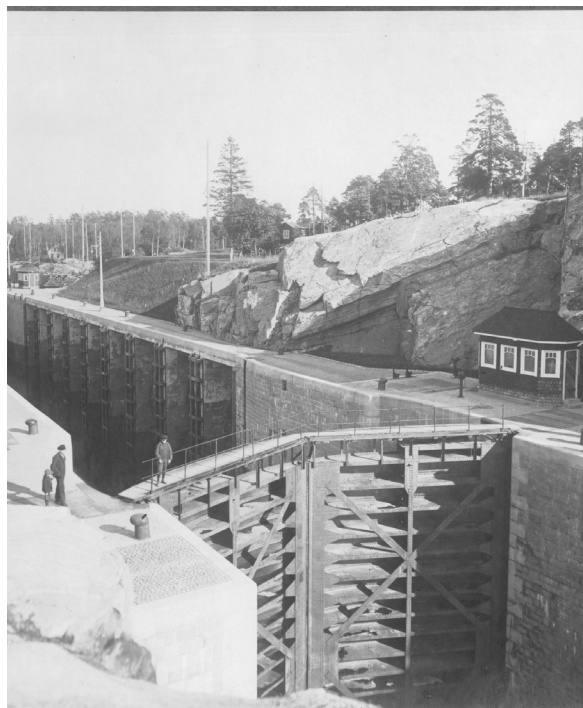
Figur 45. Del av 1916 års slussanläggning. Vid varje port står en manöverhytt. Foto 1916, Sjöfartsverket.
