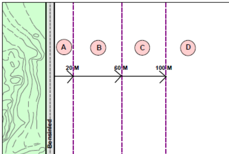
Figur 7. Skyddsavstånd från bensinled (Trollhättans Stad, 2004)
