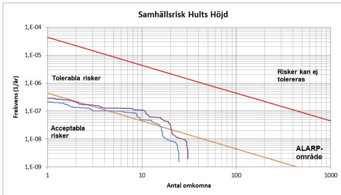
Figur 16. Samhällsrisk för transporter av farligt gods på E45. Blå linje visar ursprungsberäkningen och lila linje är osäkerhetsanalysen.
