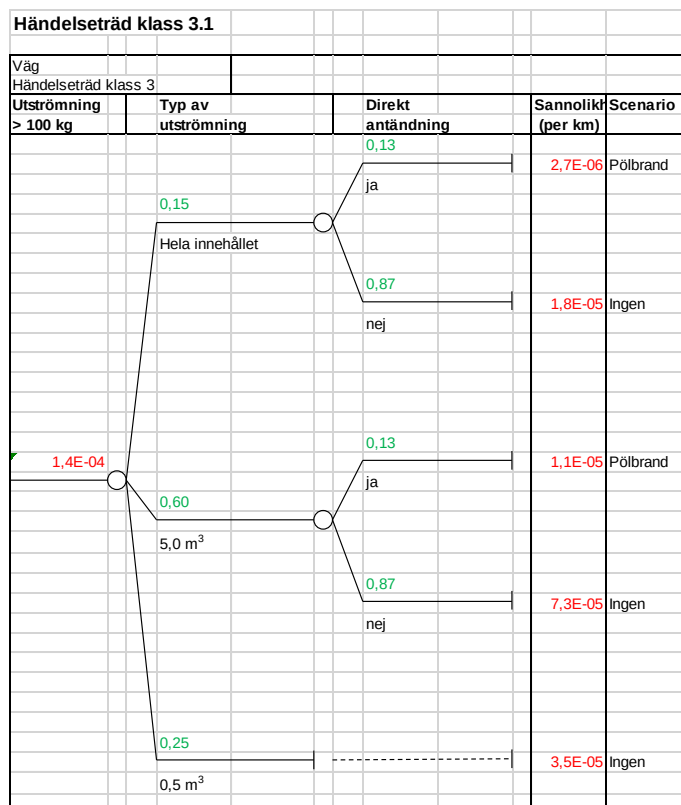
Figur 5. Händelseträd för mycket brandfarliga vätskor i klass 3.
