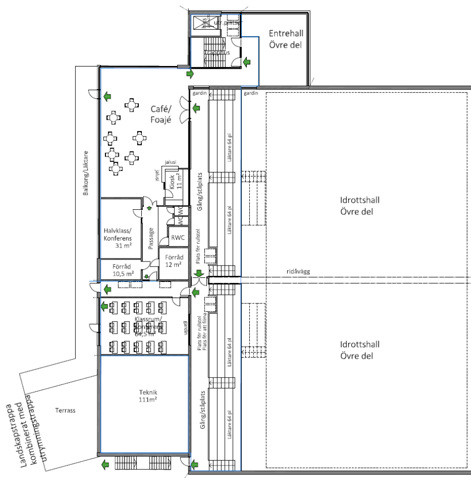
Figur 11: Planritning över idrottshallens övre plan.
