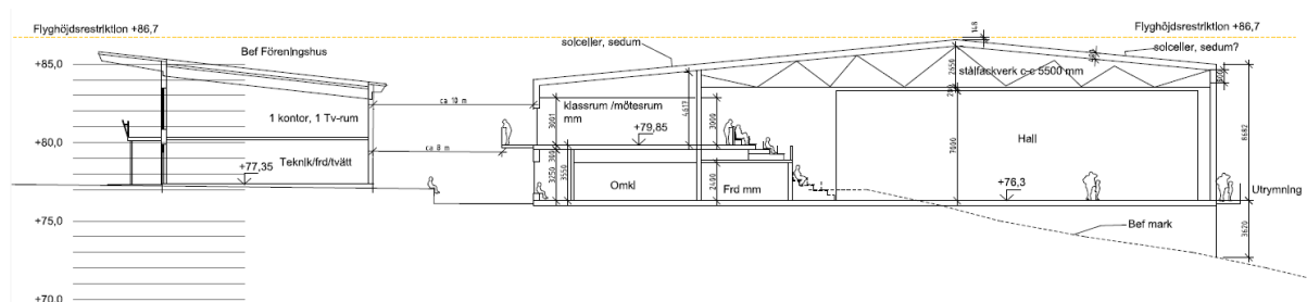
Figur 9: Sektion genom klubbstugan/fritidsgården och idrottshallen söderifrån.
