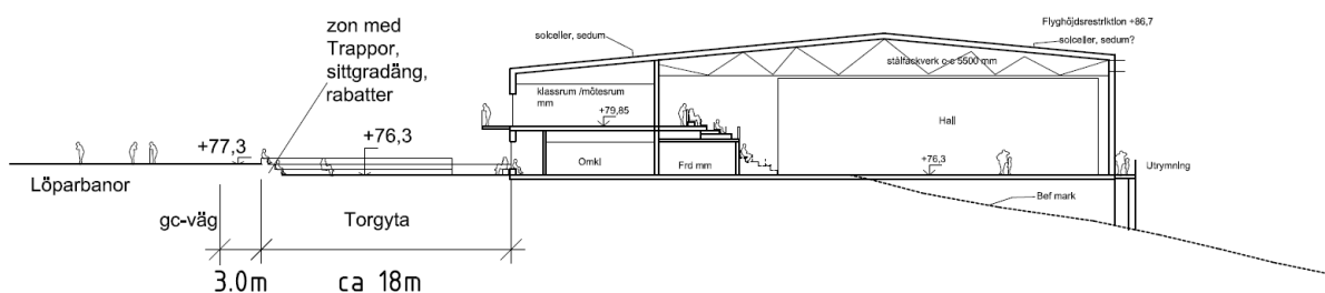
Figur 8: Sektion genom idrottshallen söderifrån.
