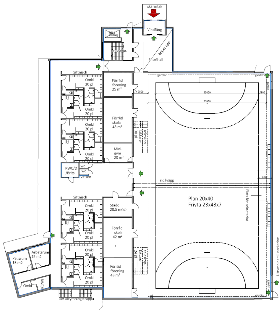
Figur 10: Planritning över idrottshallens entréplan.
