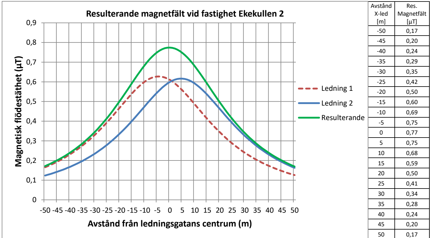
Bild ovan: Resulterande magnetfält vid beräkningstvärsnitt 1
