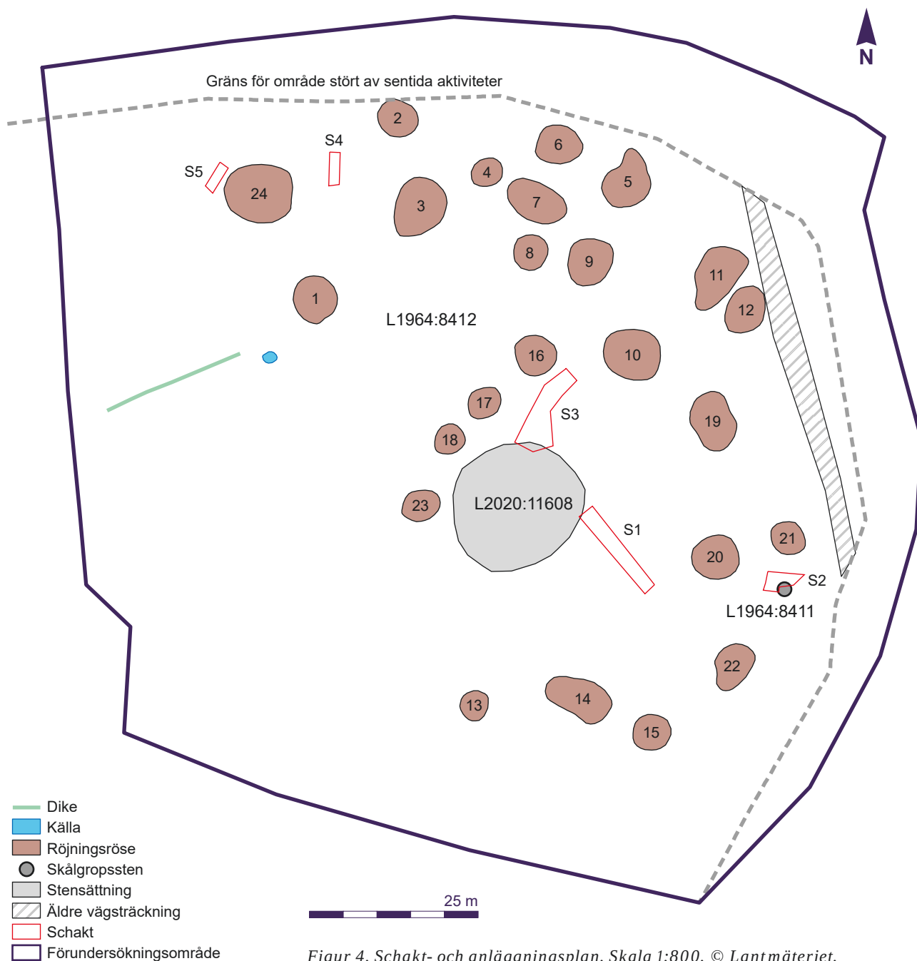
Figur 4. Schakt- och anläggningsplan. Skala 1:800. © Lantmäteriet.
